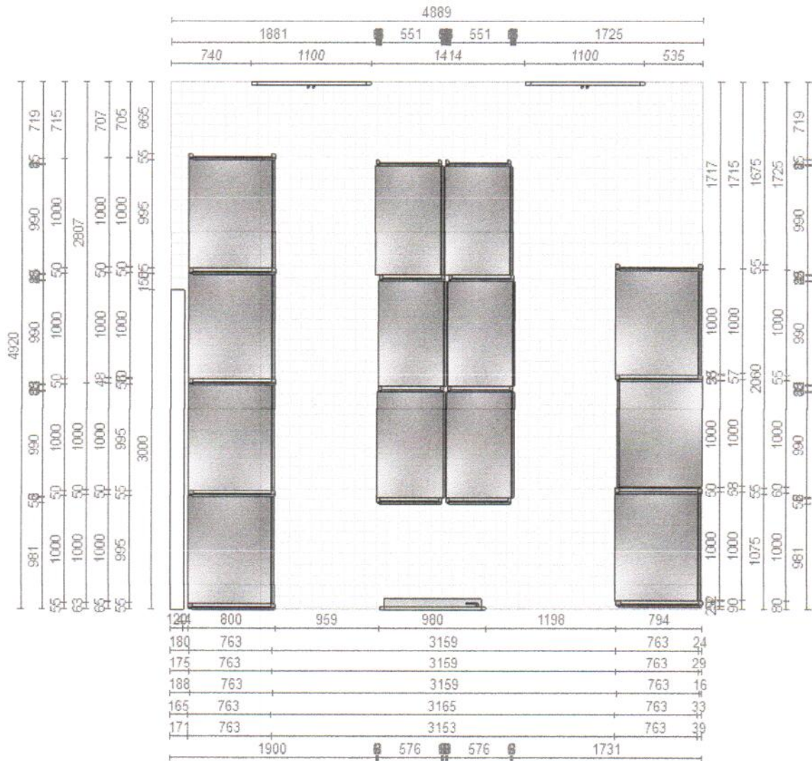
1. Схема расстановки стеллажей в помещении склада
